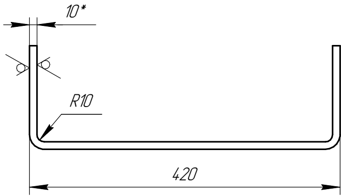
Дет. поз. 1 (1:5)
